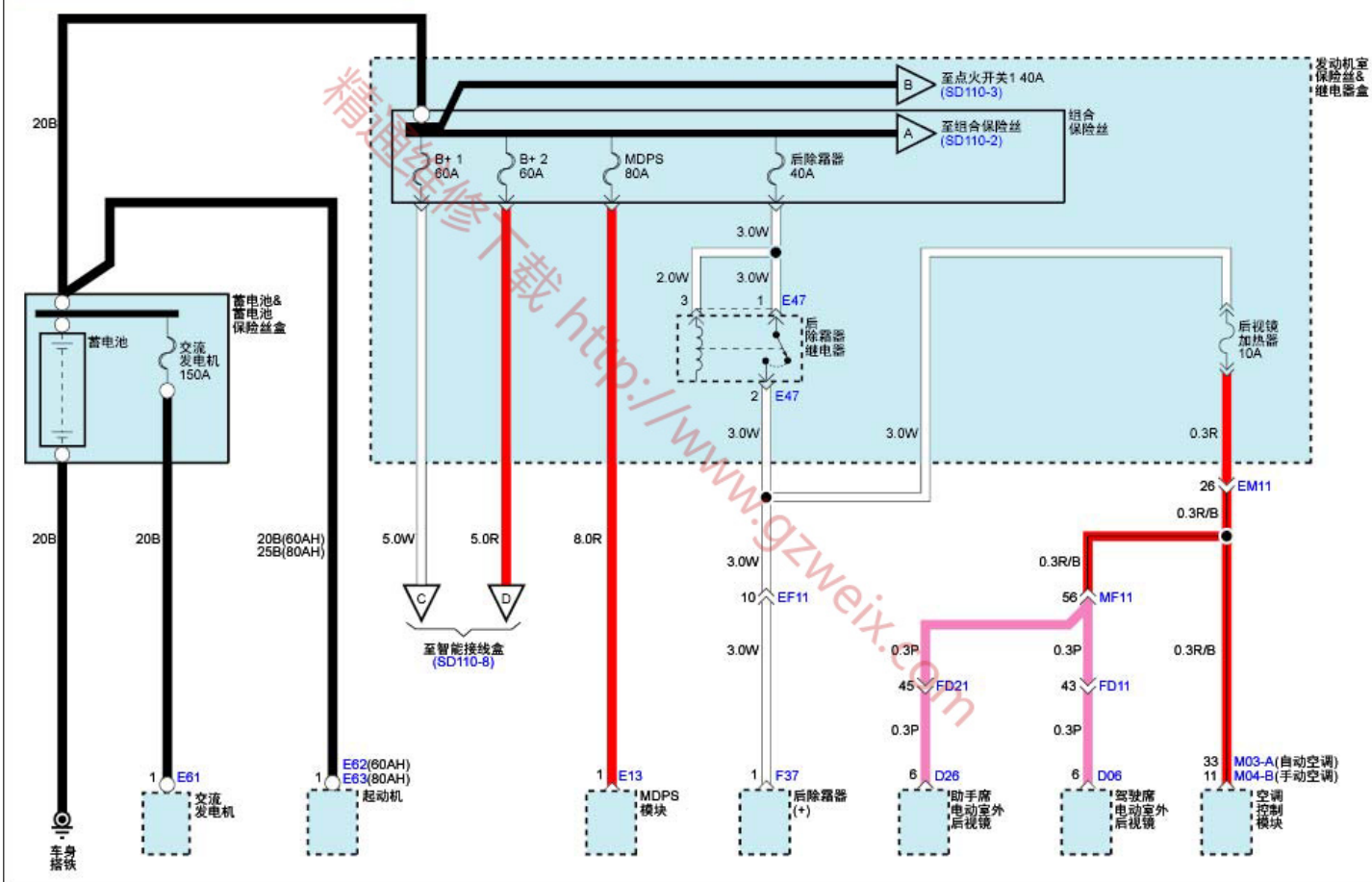
电源分布(1)
